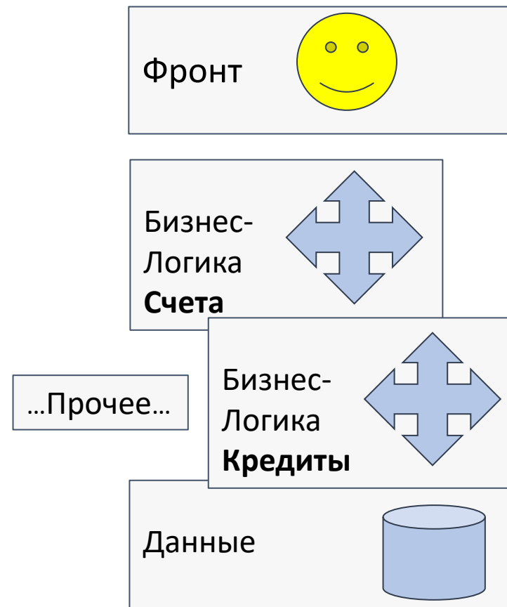
Модульная архитектура
