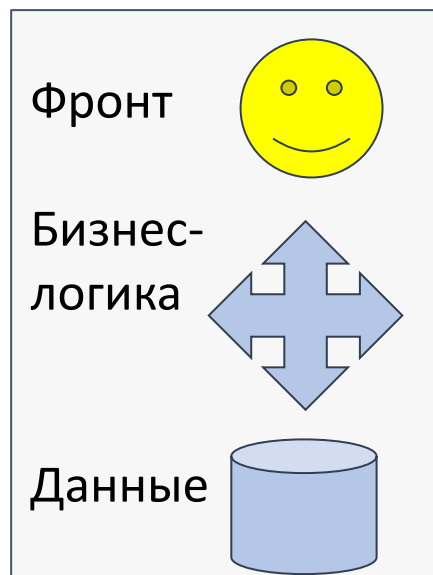
Монолит Клиент-сервер
